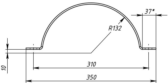
Поз.3 (Полухомут)
