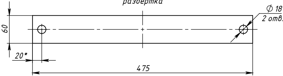
Поз.3 (Полухомут) развертка
